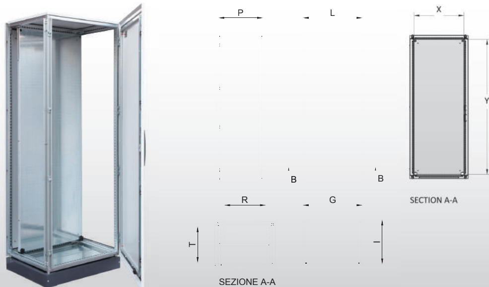
SEZIONE A-A
